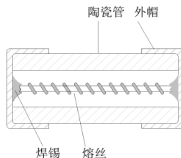
6-2 结构（焊锡耐温300℃） / Structure（Solder temperature resistance: 300℃）
